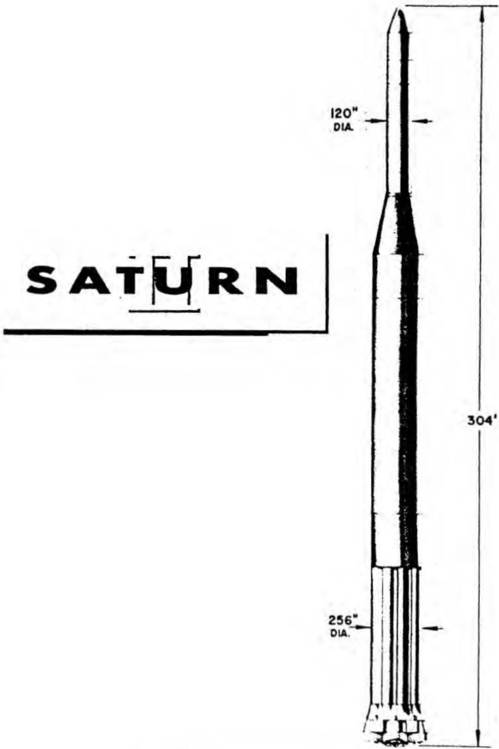
Fig. I-10. SATURN II
