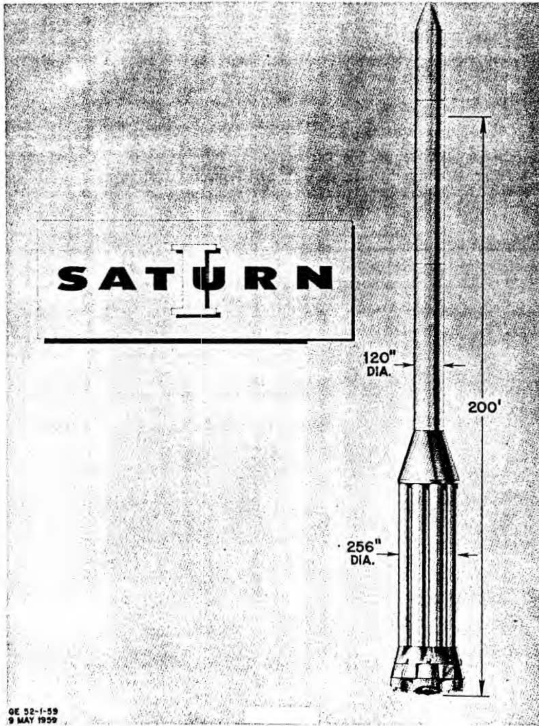
Fig. I-8. SATURN I
